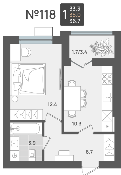
Планировка
