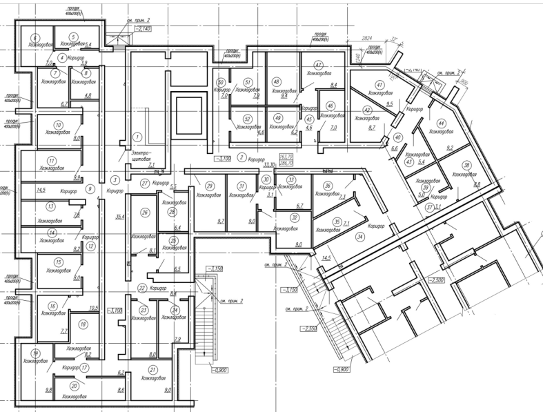
Планировка
