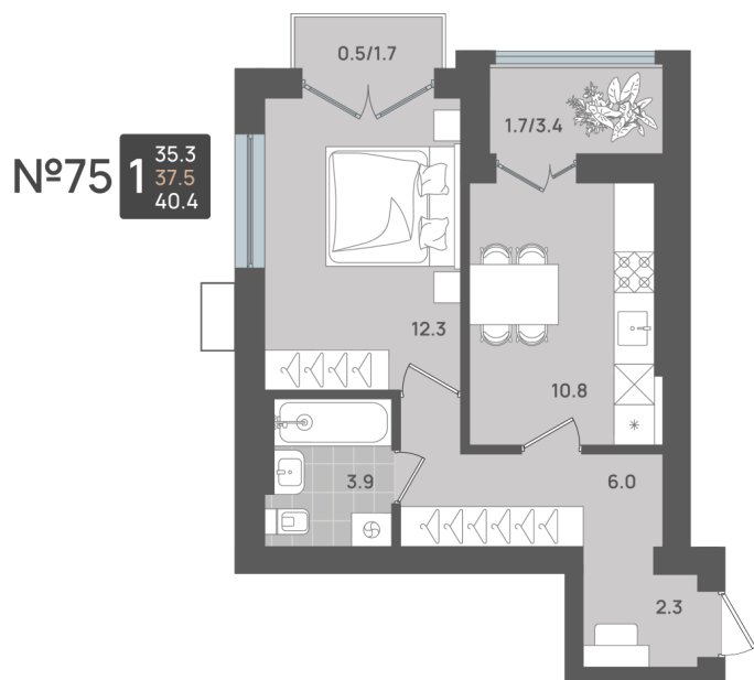
Планировка
