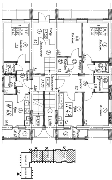
Планировка
