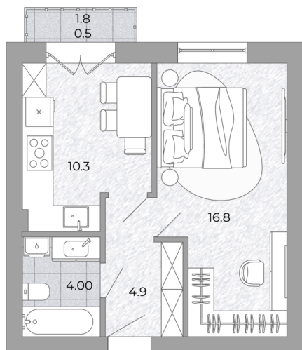
Планировка
