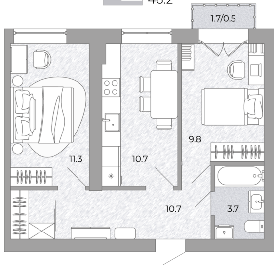
Планировка
