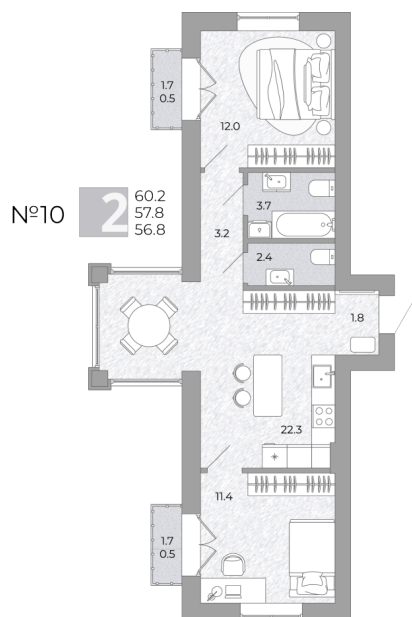
Планировка
